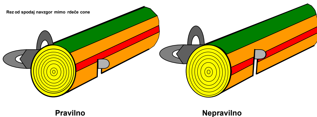
Slika 24: Prerezovanje rdeče cone od zgoraj
