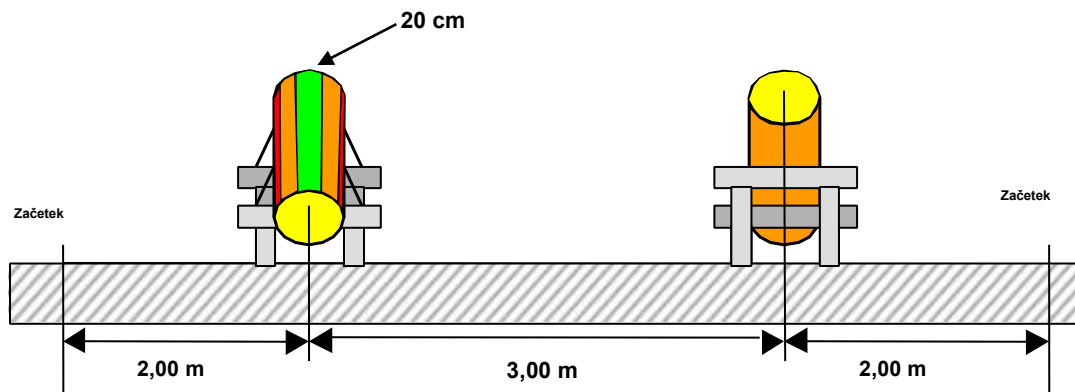
Slika 19: Postavitev hlodov za kombinirani rez
