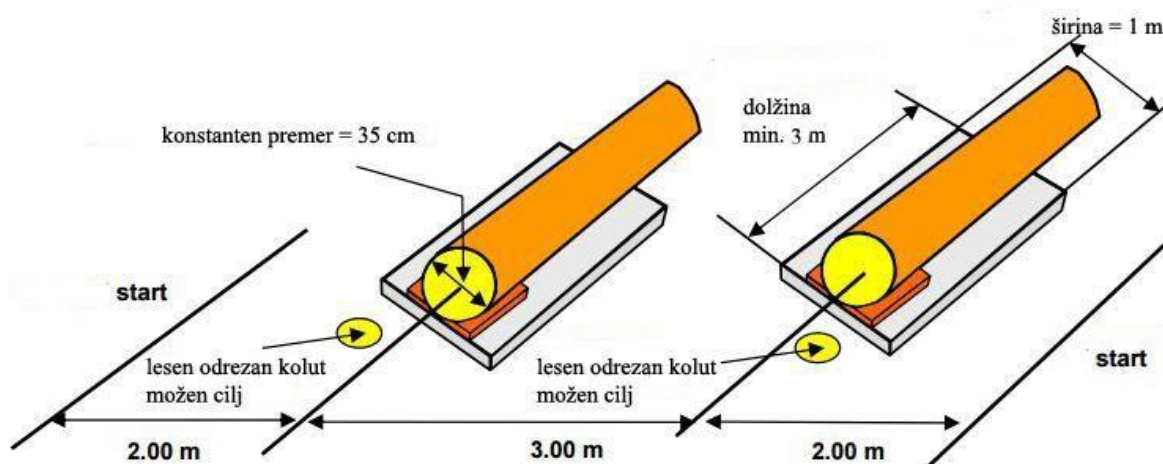
Slika 28: Pravilna postavitev opreme in hlodov pri preciznem rezu
