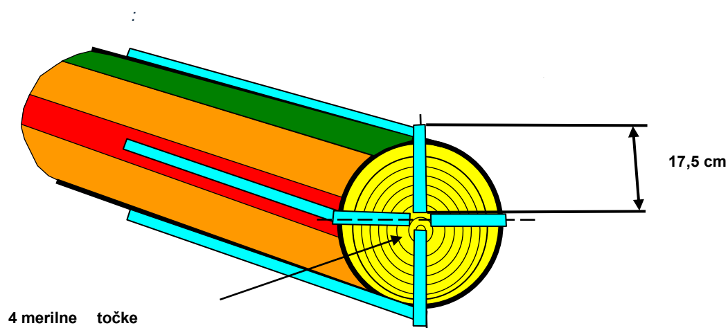
Slika 20: Meritve kotov in dolžine merilnika
