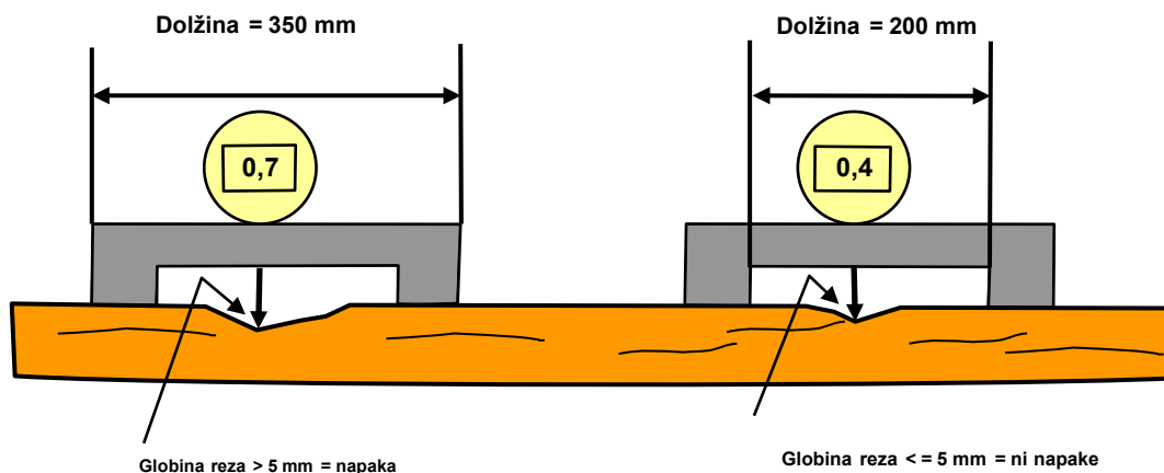
Slika 40: Poškodba debla zaradi pregloboko odrezanih vej in dolžina merilne opreme
