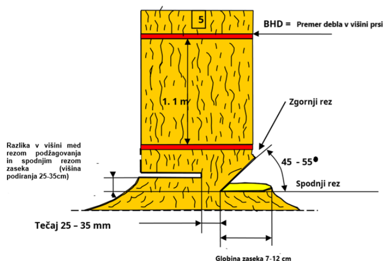
Slika 7: Mere in oznake
