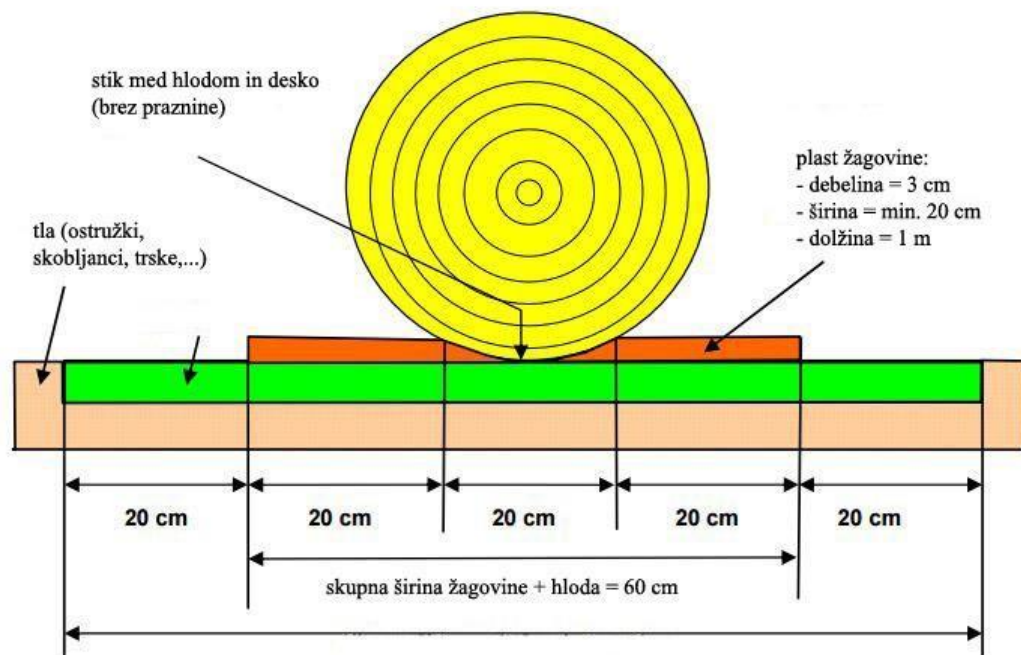
Slika 29: Položaj debla, podlage in mere plasti žagovine
