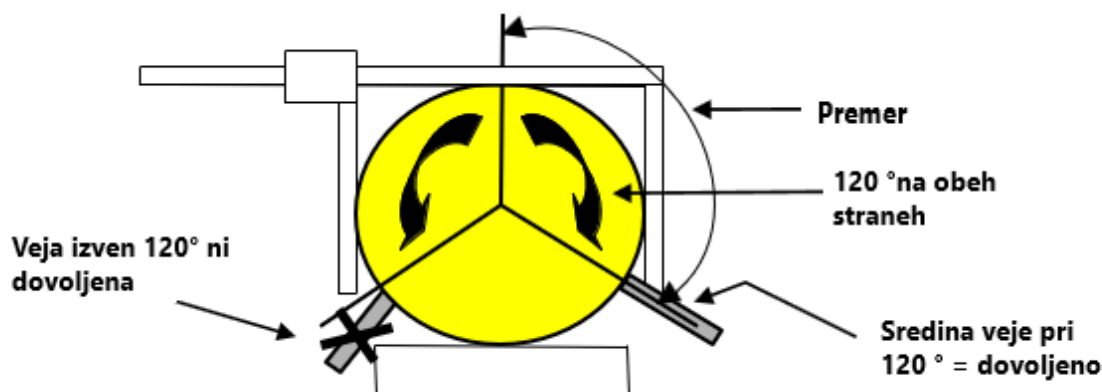
Slika 36: Območje, kleščenja levo in desno 120° (ustreza premeru debla)
