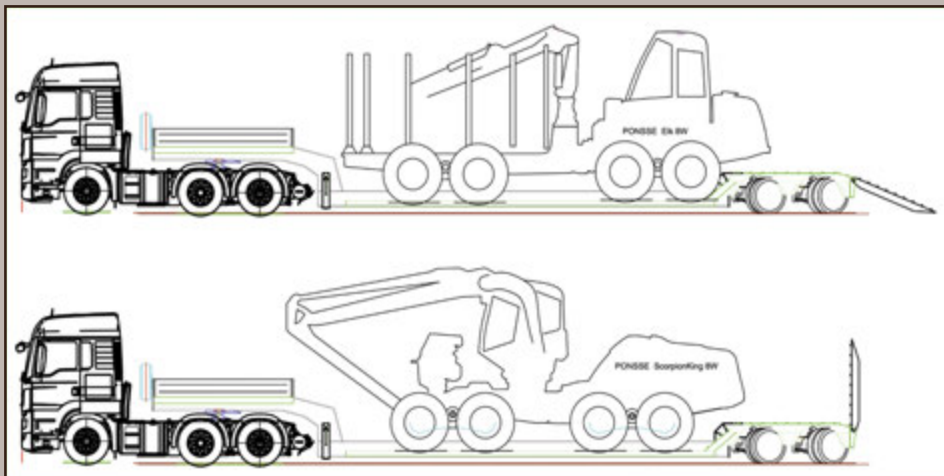
Slika 2: Skica kompozicije za transport stroj-
